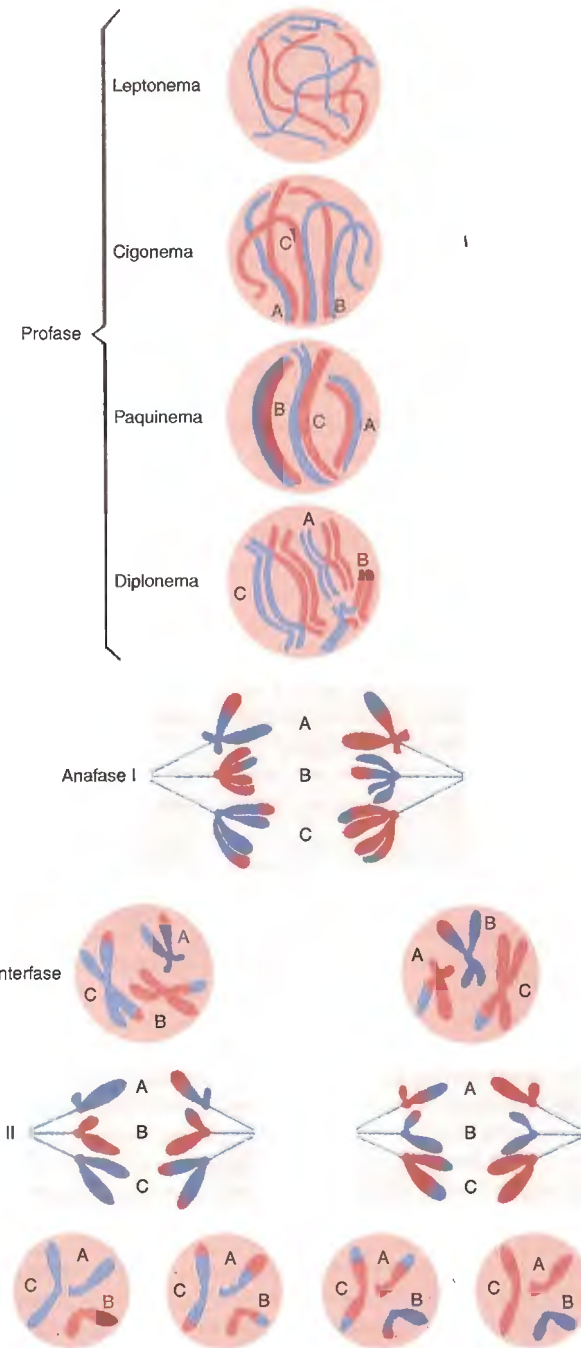
Fig. 19-2. Esquema general de la meiosis, que ilustra el apareamiento de los cromosomas homólogos, el intercambio de algunos de sus segmentos y la segregación de los cromosomas. Los cromosomas procedentes de cada progenitor están representados en azul y en rojo, respectivamente.
