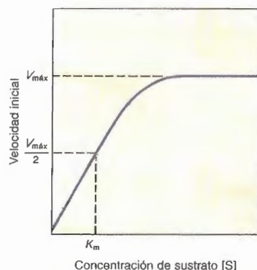
Fig. 2-34. Diagrama de la velocidad de reacción de una enzima a concentraciones de sustrato cada vez mayores. En el texto se describen la V_{\max} y la K_m . La curva es una hipérbola cuya primera parte sigue una cinética de primer orden (es decir, la reacción es proporcional a la concentración del sustrato); la segunda parte corresponde a la saturación, que tiene una cinética de orden cero (ya que no depende de la concentración del sustrato).
