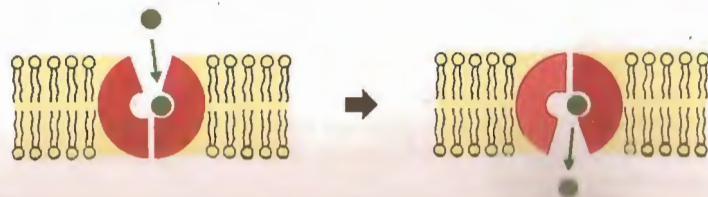
Fig. 3-24. Esquema que representa a una permeasa y el modo como la atraviesan los solutos.
