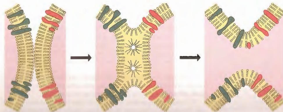
Fig. 3-13. Esquema que ilustra el posible mecanismo molecular responsable de la fusión de dos membranas celulares. (De R. Schaier y P. Overath.)
