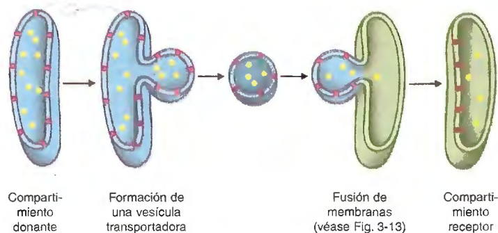
Fig. 7-2. Esquemas secuenciales que ilustran la formación de una vesícula en la membrana de un compartimiento donante y la fusión de la membrana vesicular con la membrana del compartimiento receptor.
