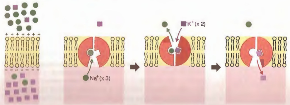
Fig. 3-26. \text{Na}^+\text{K}^+ -ATPasa o bomba de \text{Na}^+\text{K}^+ .
