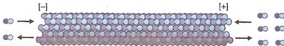
Fig. 5-6. Polimerización (alargamiento) y despolimerización (acortamiento) de los microtúbulos por sus dos extremos.
