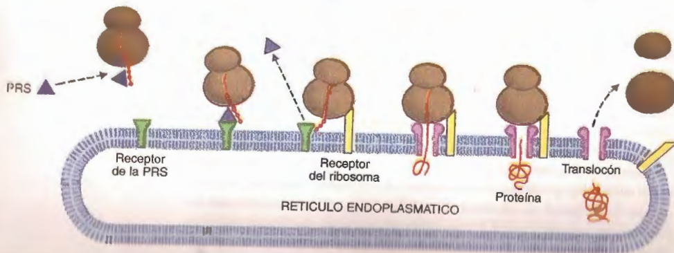
Fig. 7-9. Unión del ribosoma con la membrana del RER. Obsérvese el receptor de la PRS, el receptor del ribosoma y el paso de la proteína a través del translocón.
