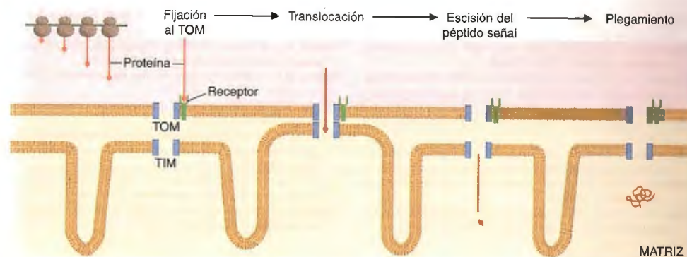
Fig. 8-20. Modo como ingresa en la matriz mitocondrial una proteína procedente del citosol.
