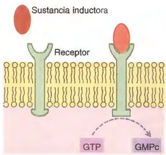
Fig. 11-6. Receptor membranoso cuyo dominio citosólico posee actividad de guanilato ciclasa.
