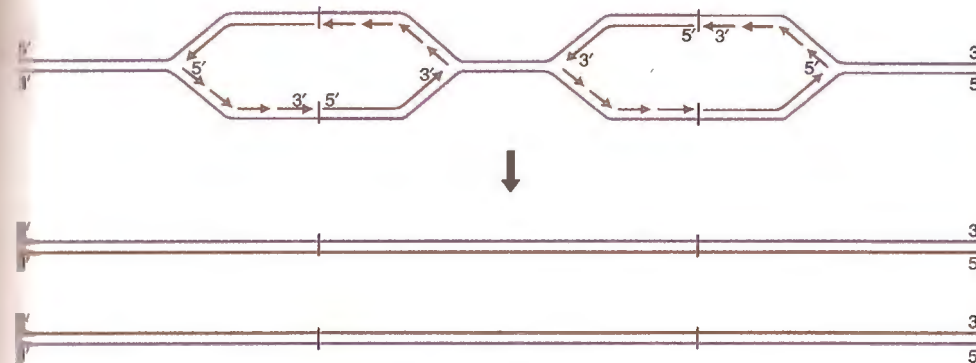
Fig. 17-9. Esquema que muestra dos replicones contiguos y los lugares donde se origina la replicación. Asimismo muestra el carácter bidireccional de la replicación y los sectores donde el ADN se sintetiza en forma continua y discontinua.
