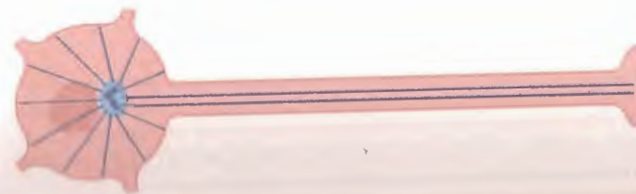
Fig. 5-13. Distribución de los microtúbulos en la neurona.
