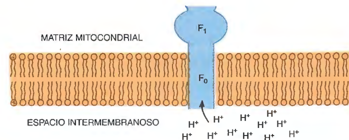
Fig. 8-13. Representación de la ATP sintasa en la membrana mitocondrial interna.
