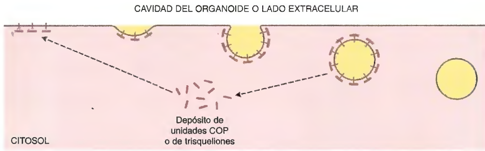
Fig. 7-32. Evolución seguida por la membrana durante la formación de una vesícula. Se ilustra también la dinámica de las unidades COP y de los triqueliones.
