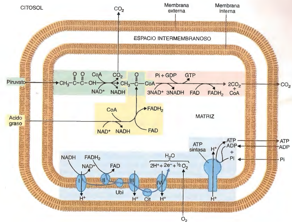
Fig. 8-10. Representación gráfica de la mitocondria. Se ilustran las reacciones correspondientes a la descarboxilación oxidativa (verde), al ciclo de Krebs (rojo), a la \beta -oxidación de los ácidos grasos (amarillo) y a la fosforilación oxidativa (azul). La acetil CoA deriva tanto de la descarboxilación oxidativa como de la \beta -oxidación de los ácidos grasos y es el punto de partida del ciclo de Krebs. I, NADH deshidrogenasa; II, Succinato deshidrogenasa (y FAD); Ubi, Ubiquinona ; b-c 1 , Complejo b-c 1 ; Cit, Citocromo c ; IV, Citocromo oxidasa .
